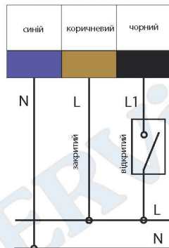
Схема електричного підключення
